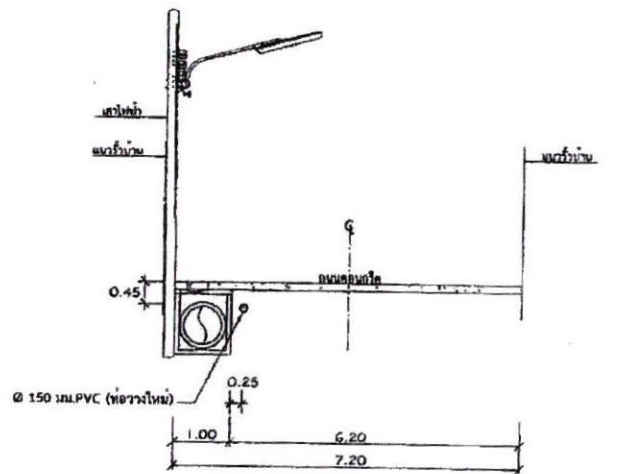
รูปตัด ก - ก 1 : 100
