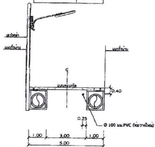
รูปตัด ก - ค 1 : 100
