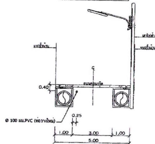
รูปตัด ง - ง 1 : 100
