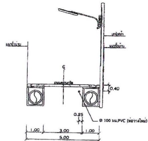
รูปตัด ข - ข 1 : 100
